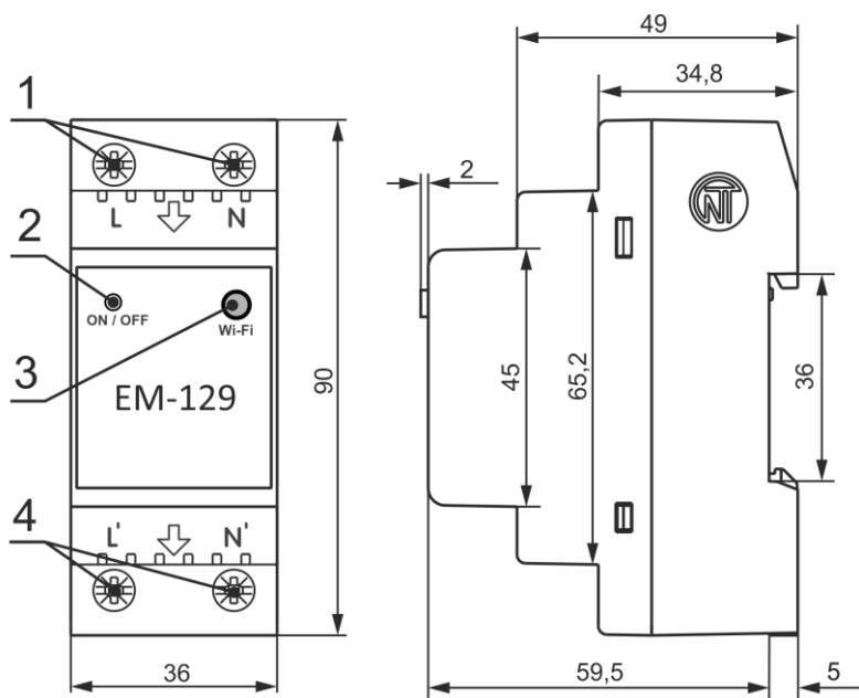
Рисунок 1 – Органы управления, габаритные и установочные размеры EM-129
