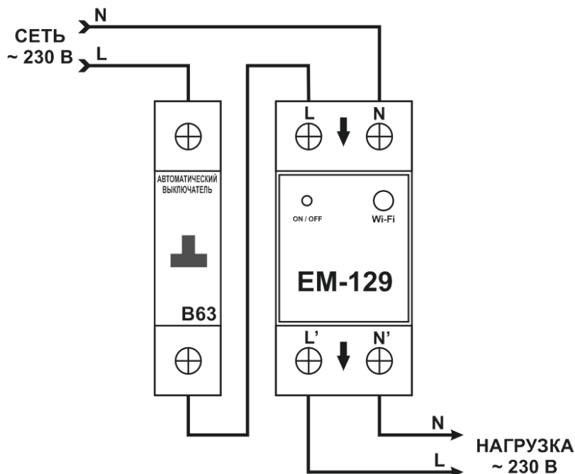
Рисунок 2 – Схема подключения EM-129
